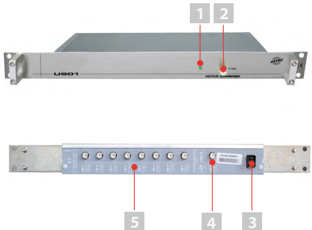
Bild 1: U 901 Zusammenführungsnetzwerk (Frontseite des VZN 8 entspricht der Rückseite des U 901)
